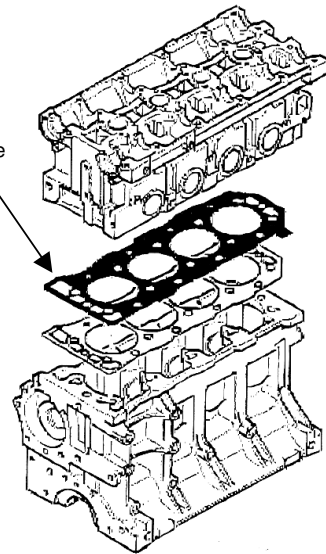
Abb 1. Verbauen Sie die Zylinderkopf-Zwischenlage mit der schwarz beschichteten Seite in Richtung Zylinderkopf.
